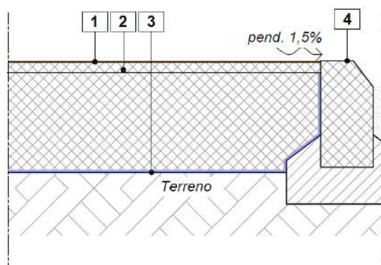
Scheda tecnica cordolo in cls
