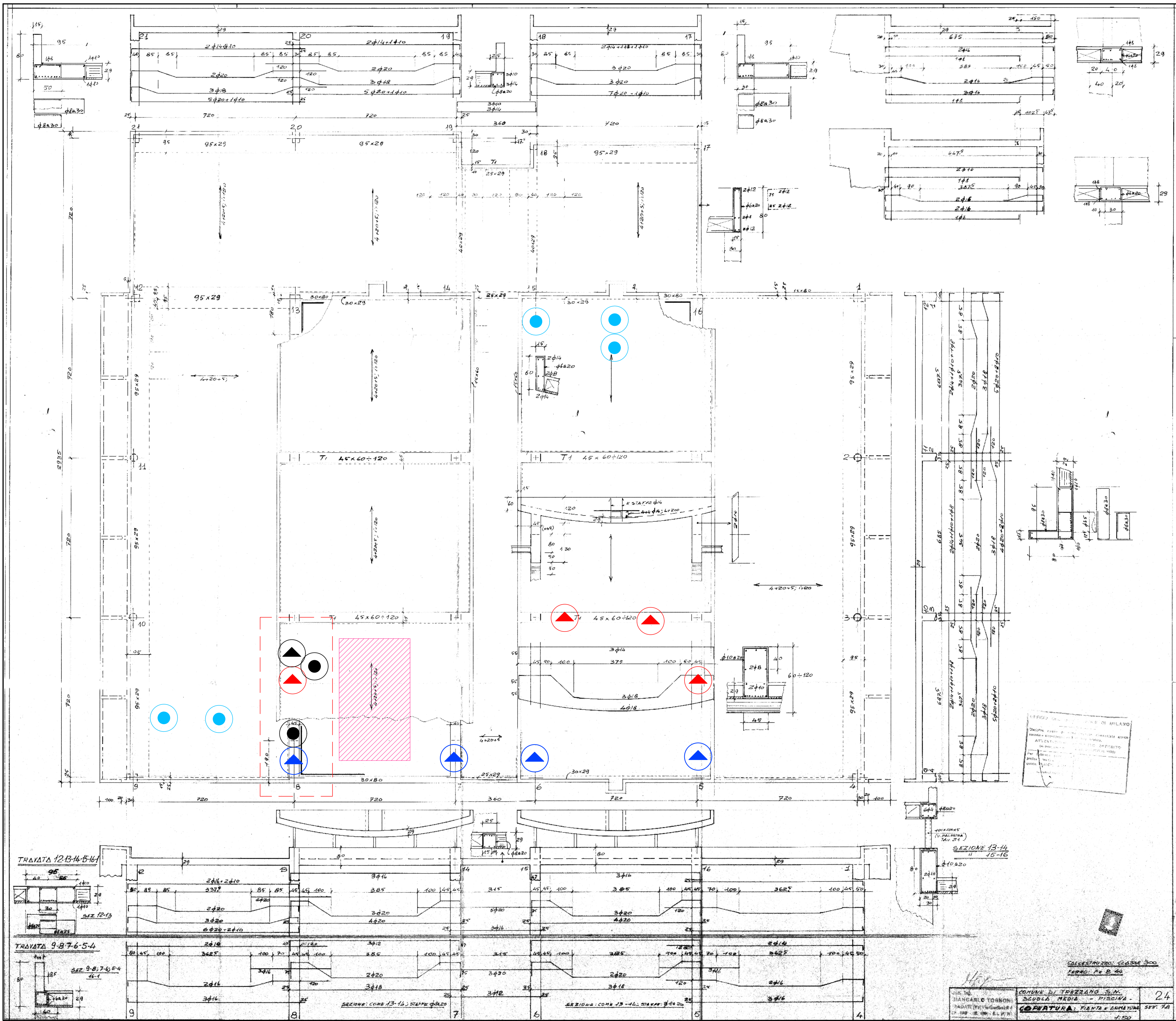
TAV. 24 - PIANTE COPERTURA PISCINA
