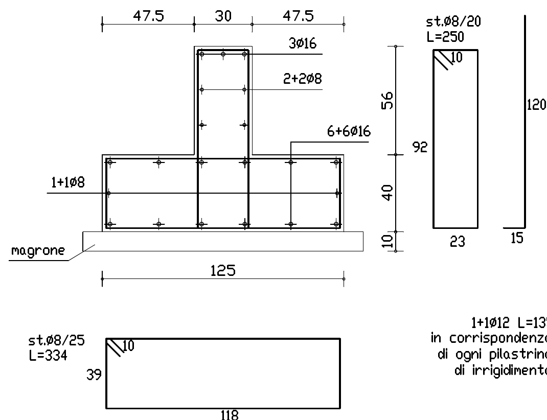
SEZIONE A-A (1:20)
