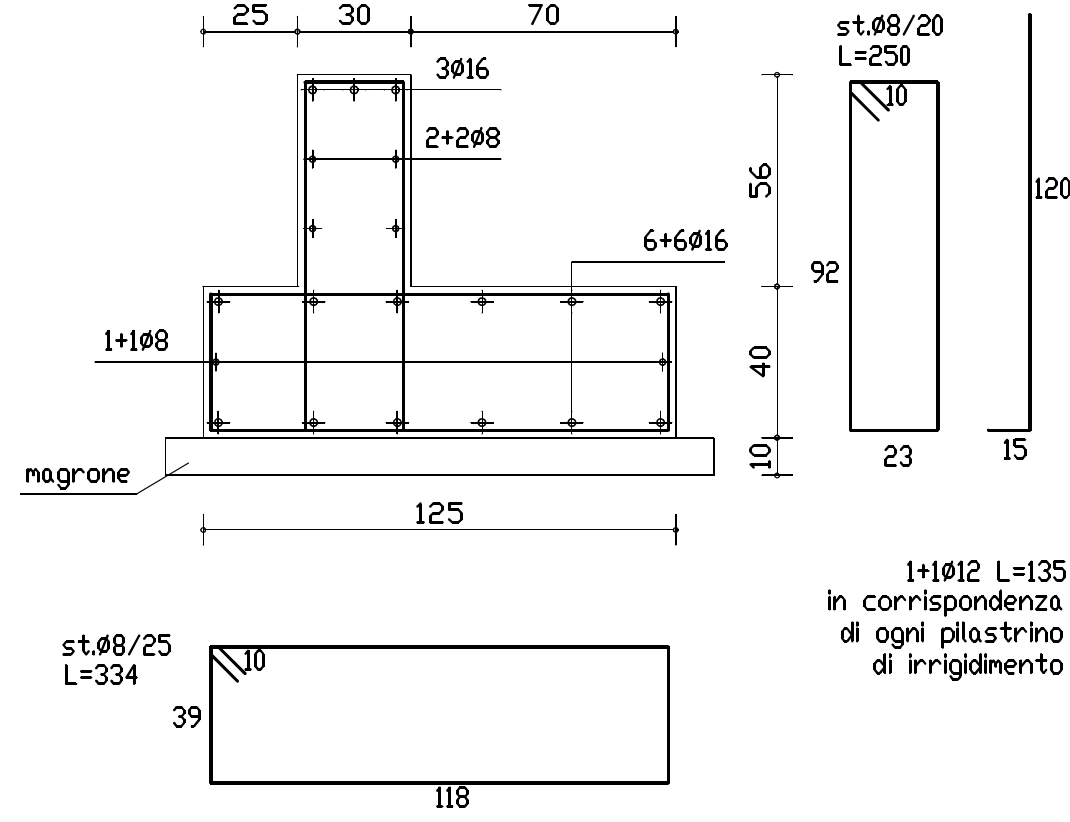
SEZIONE B-B (1:20)
