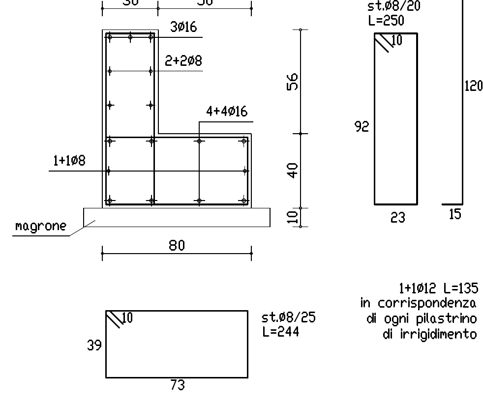
SEZIONE C-C (1:20)
