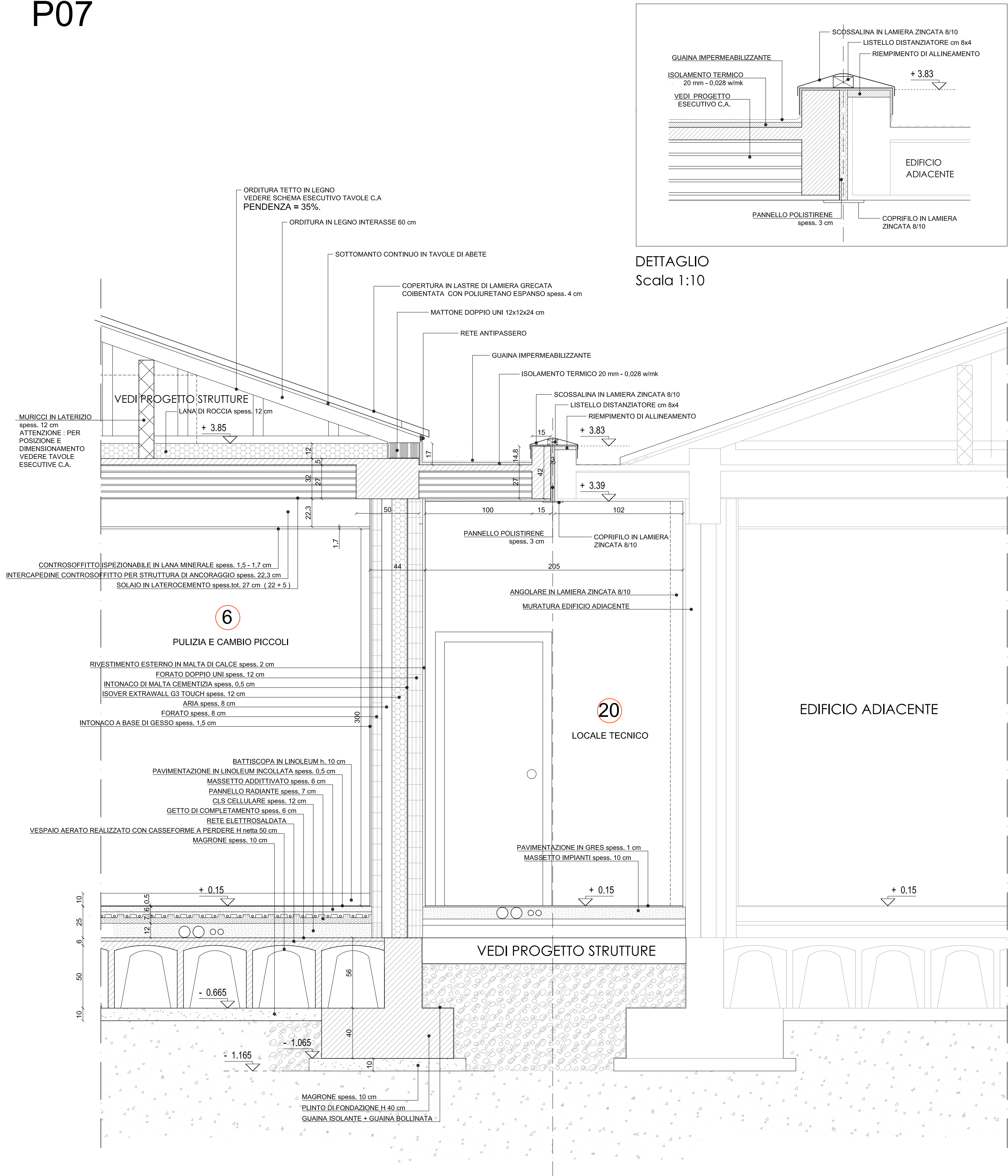
SEZIONE VERTICALE - P07 DETTAGLIO - scala 1:20
